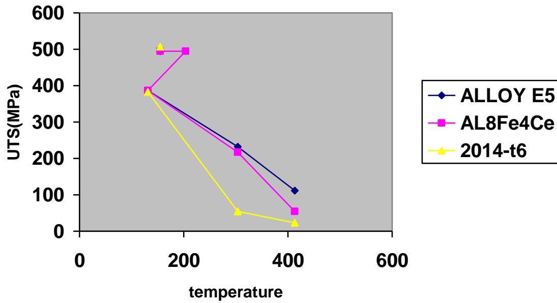
High Temperature Strength of i/m ۲۰۱۴-t۶ and Experimental and Al 8 Fe 4 Ce Alloy E5 متالورژی پودر
